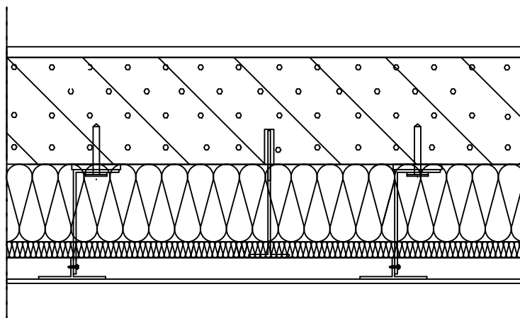
SNITT DETALJ A-A
