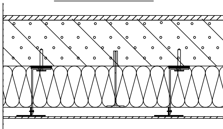
SNITT DETALJ A-A
