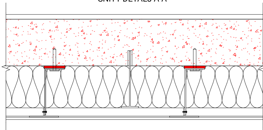
SNITT DETALJ A-A
