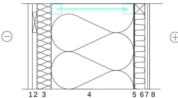
DETALJE SEKTION A-A
