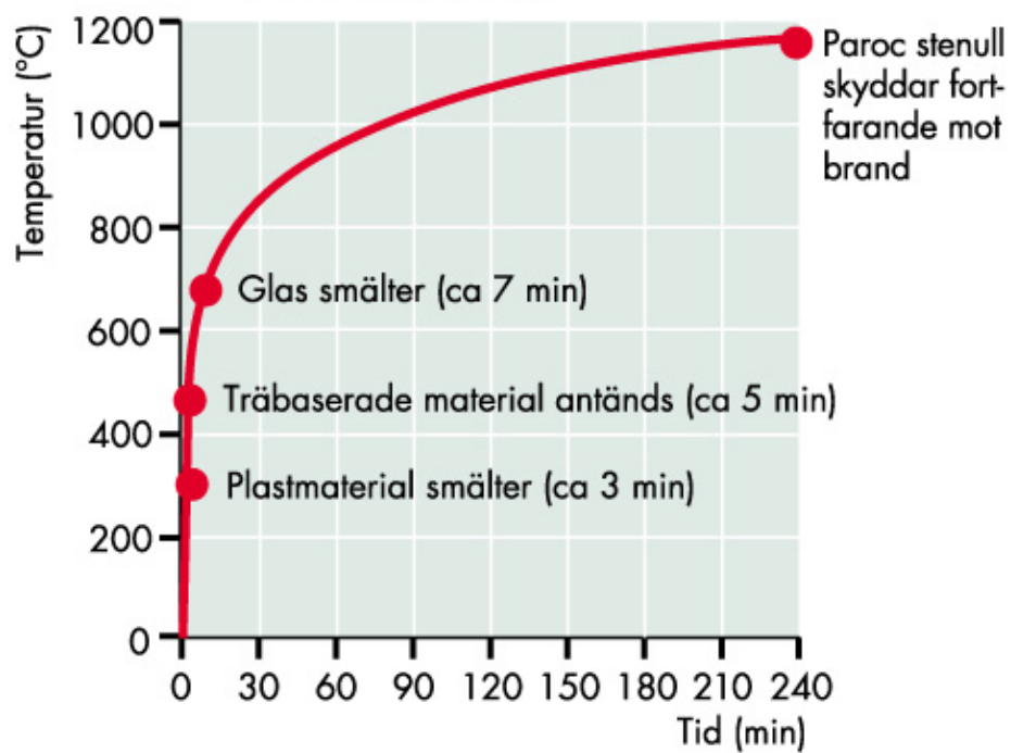
Standardbrandkurva
