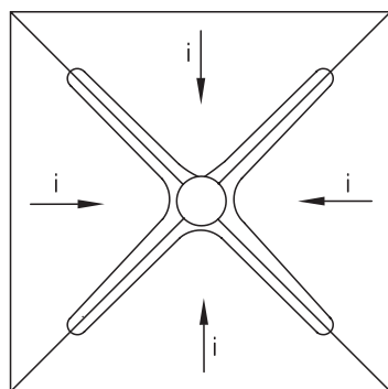
Šildymo kabelių klojimo schema plane
