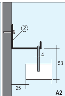
Detalji A2: ripustus seinästä
