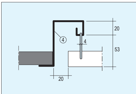
Detalji C: ripustus kiinteästä alakatosta
