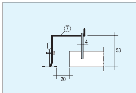
Detalji F: ripustus alakaton kannatinlistoista
