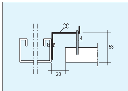
Detalji B: ripustus kaapelikourusta
