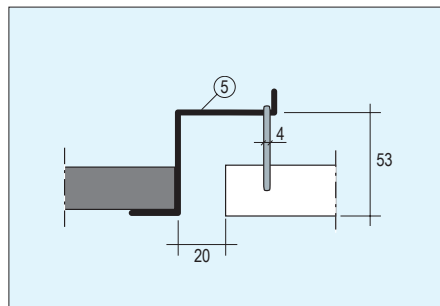
Detalji D: ripustus kiinteästä alakatosta
