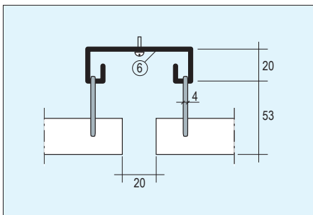
Detalji E: kaksoisripustus
